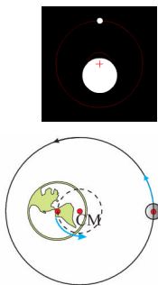
Slika 5.2: Kretanje Zemlje i Meseca oko zajedničkog centra masa.
